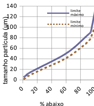
Distribuição Granulométrica e Ciclo de Estufagem
